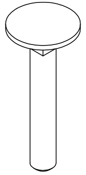
DIN 603 M8x45 x20
